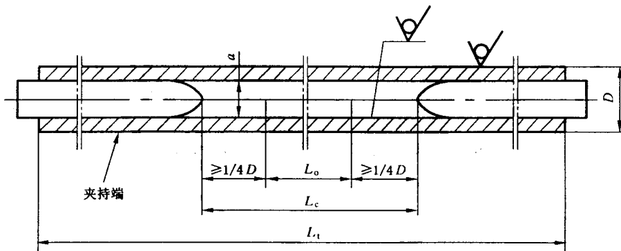
图 D1 管段试样的塞头位置
