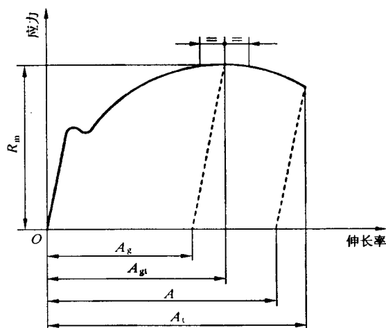
图1 伸长的定义
